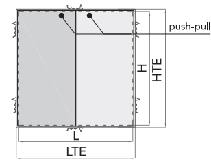
TELAIO 4 LATI ANTA DOPPIA
