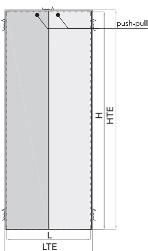
TELAIO 3 LATI ANTA DOPPIA
