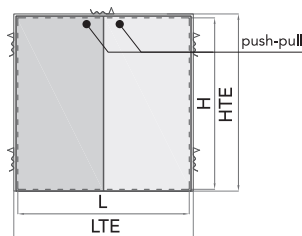
TELAIO 3 LATI ANTA DOPPIA
