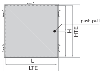
TELAIO 3 LATI ANTA SINGOLA
