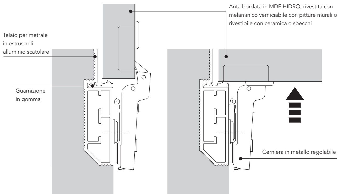
Chiusura Push-Pull di serie
