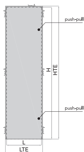
TELAIO 3 LATI ANTA SINGOLA
