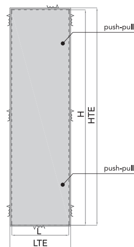
TELAIO 4 LATI ANTA SINGOLA
